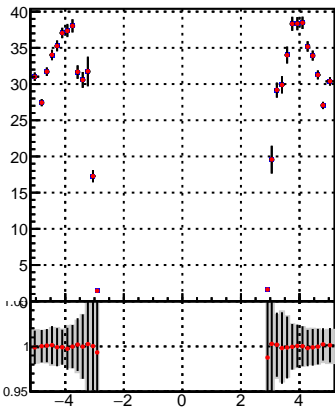
p_offset_eta_np30_hfh
