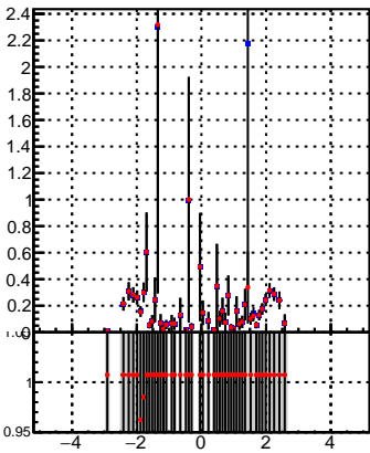
p_offset_eta_np30_lep
