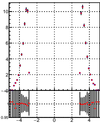
p_offset_eta_np30_hfe
