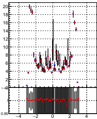
p_offset_eta_np30_chu
