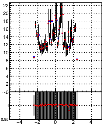
p_offset_eta_np30_chm
