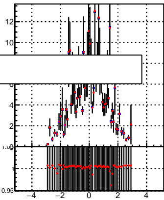
p_offset_eta_np30_ne
