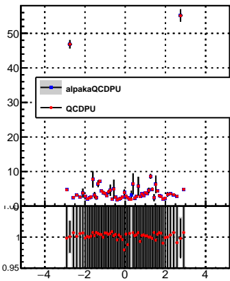
p_offset_eta_np30_nh
