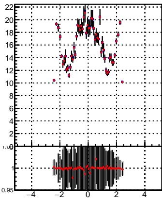
p_offset_eta_npv37_chm
