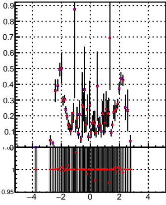
p_offset_eta_npv37_lep
