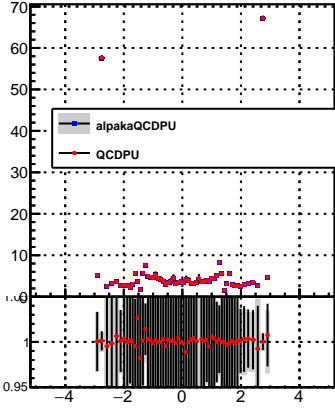
p_offset_eta_npv37_nh
