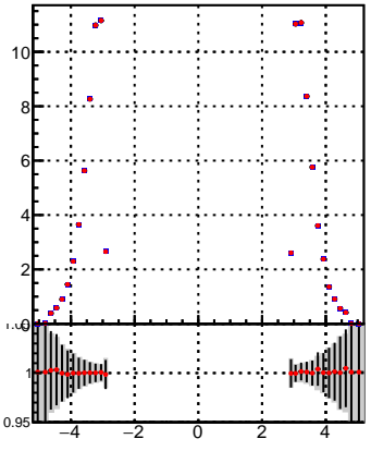
p_offset_eta_npv37_hfe
