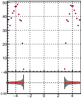
p_offset_eta_npv37_hfh
