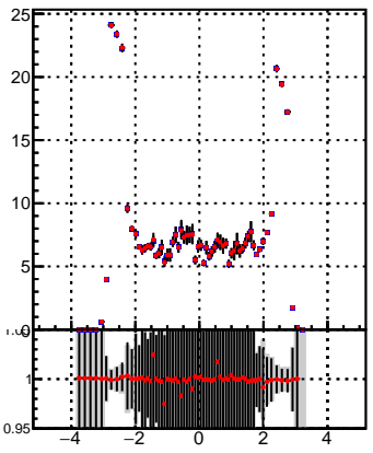
p_offset_eta_npv37_chu
