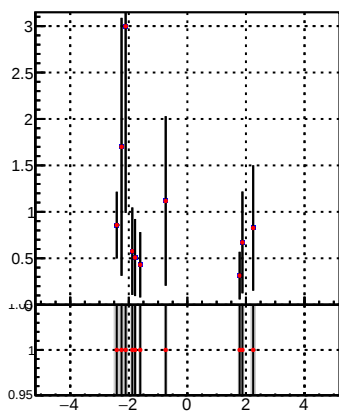
p_offset_eta_npv83_lep
