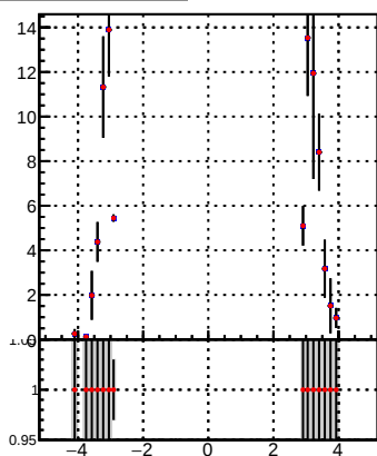
p_offset_eta_npv83_hfe
