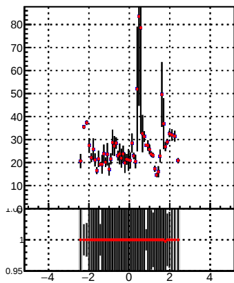
p_offset_eta_npv83_chm
