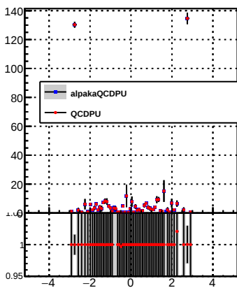
p_offset_eta_npv83_nh
