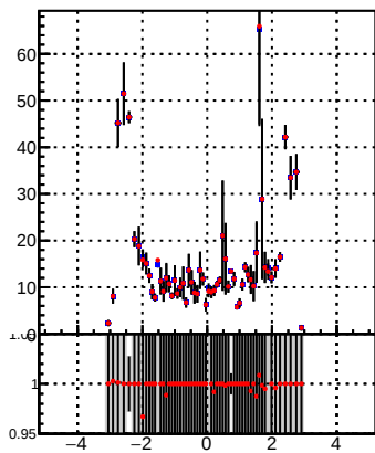
p_offset_eta_npv83_chu
