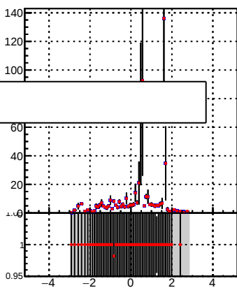
p_offset_eta_npv83_ne
