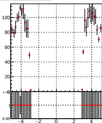
p_offset_eta_npv83_hfh
