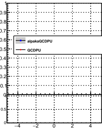
p_offset_eta_np90_nh
