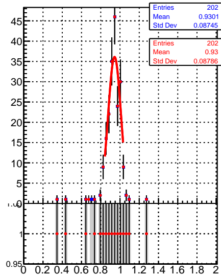
Raw Jet response (pT/pTgen) in 1032 &lt;math&gt;\leq p_t &lt; 1248, 1.3 \leq |\eta| &lt; 2.1&lt;/math&gt;
