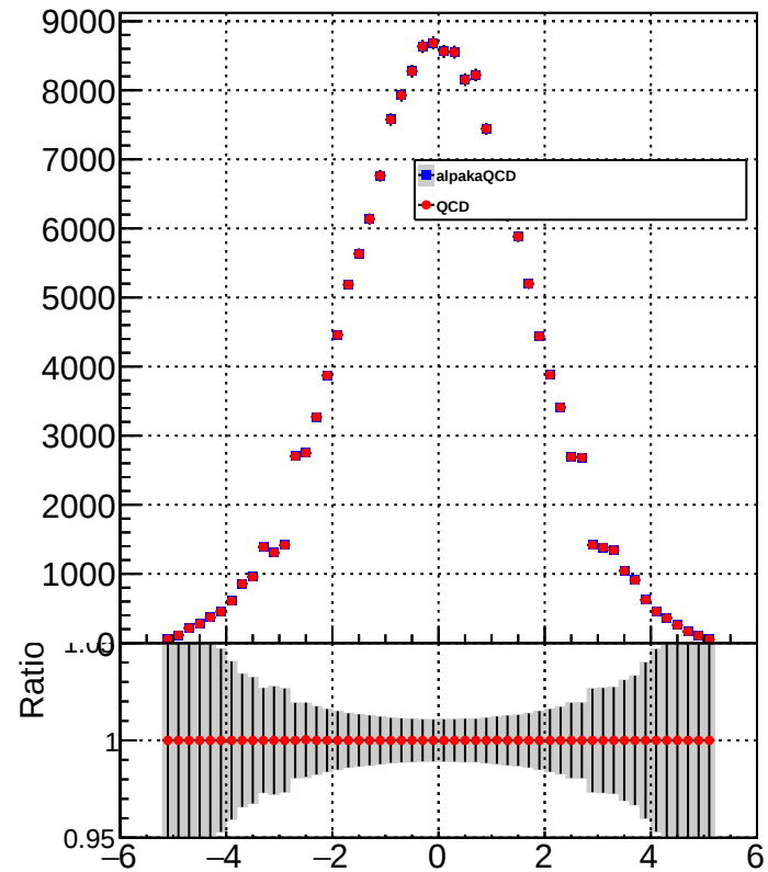
CorrJetEta Pt>20
