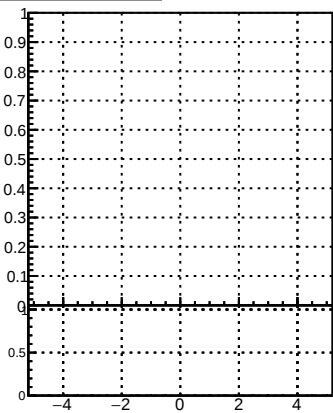
p_offset_eta_npv16_hfe
