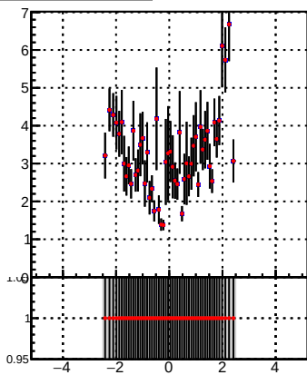
p_offset_eta_npv2_chm
