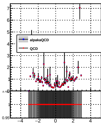
p_offset_eta_npv2_nh
