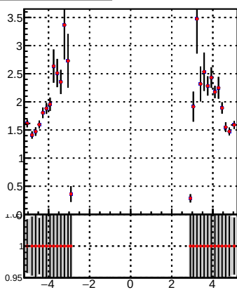
p_offset_eta_npv2_hfh
