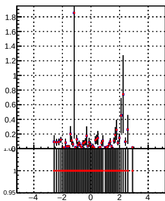
p_offset_eta_npv2_lep
