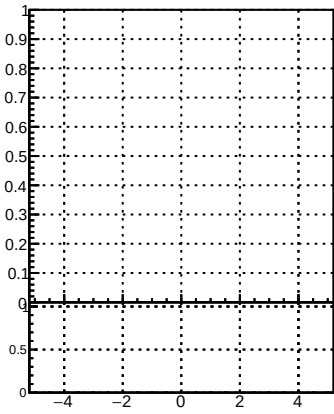
p_offset_eta_npv35_hfe
