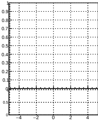
p_offset_eta_npv5_hfe
