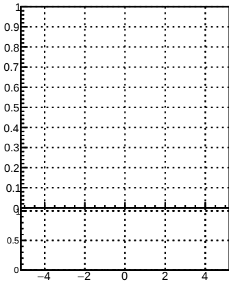
p_offset_eta_npv5_chu
