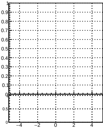
p_offset_eta_npv58_chu
