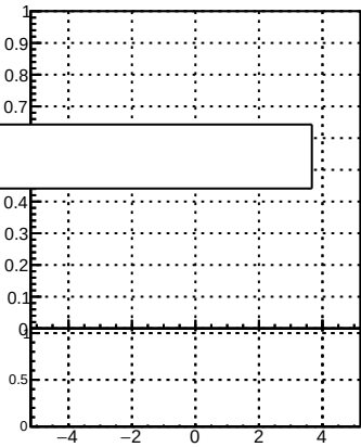
p_offset_eta_npv58_ne
