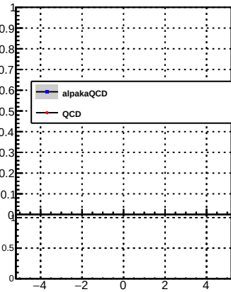
p_offset_eta_npv58_nh
