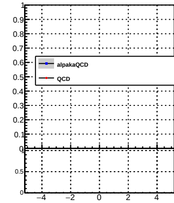
p_offset_eta_npv68_nh
