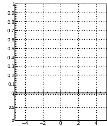
p_offset_eta_npv68_chu
