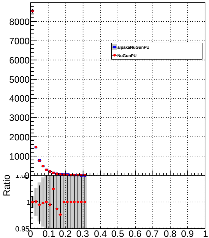
HFEMEnergyFraction
