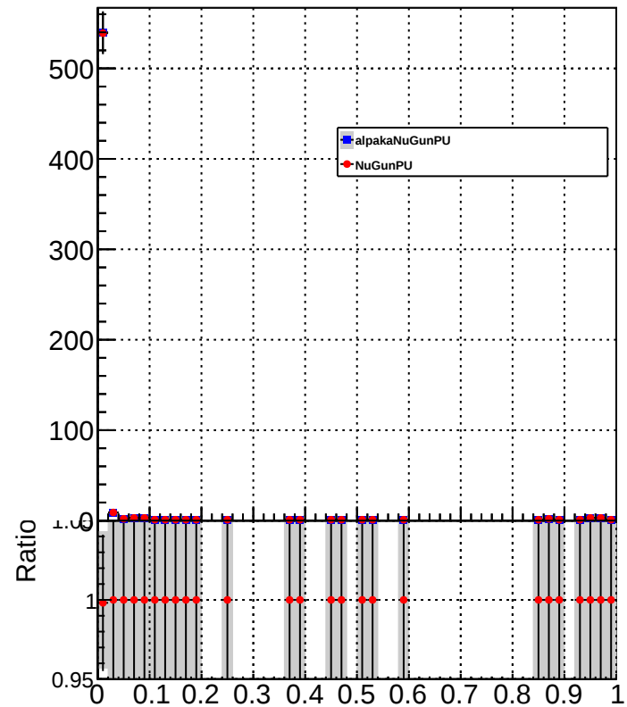
muonEnergyFraction
