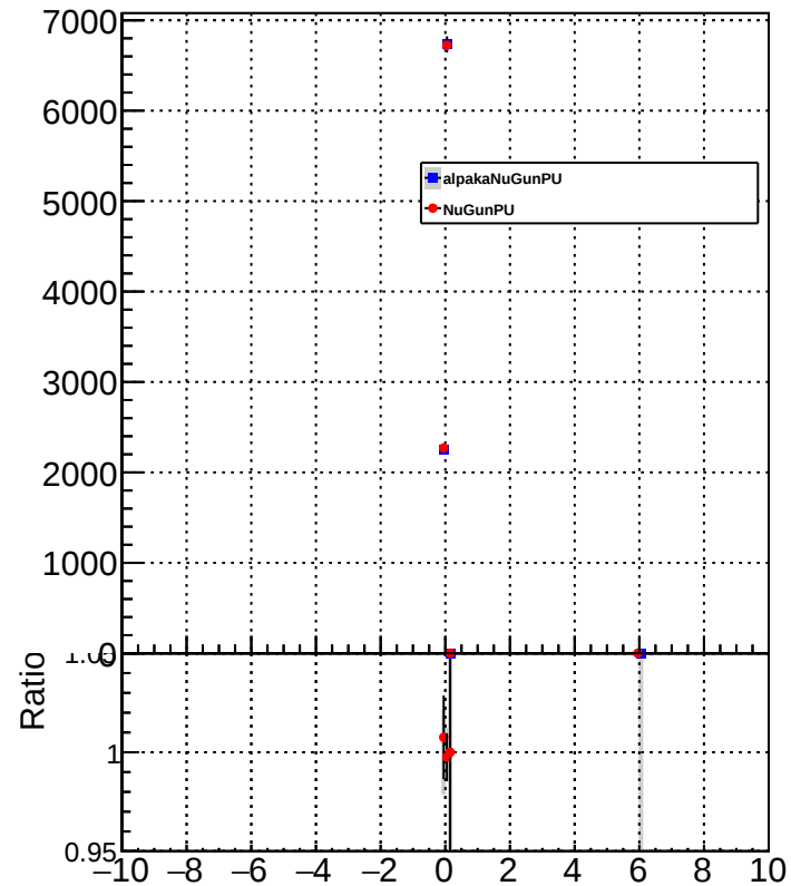
METUnc_MuonEnDown
