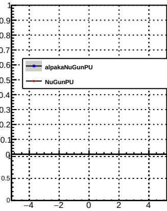
p_offset_eta_npv16_nh
