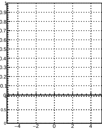
p_offset_eta_npv16_chm
