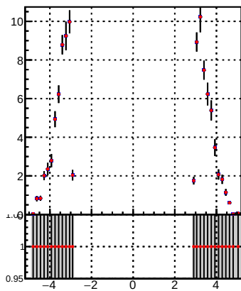
p_offset_eta_npv28_hfe
