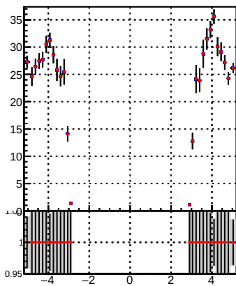
p_offset_eta_npv28_hfh
