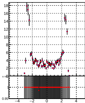
p_offset_eta_npv28_chu
