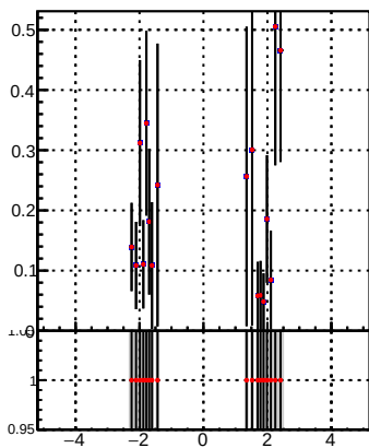
p_offset_eta_npv28_lep
