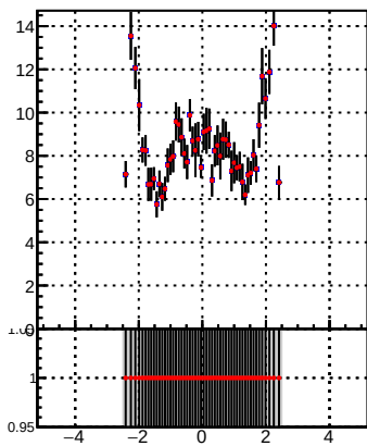
p_offset_eta_npv28_chm
