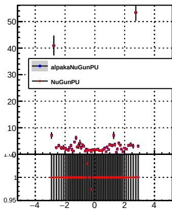
p_offset_eta_npv28_nh
