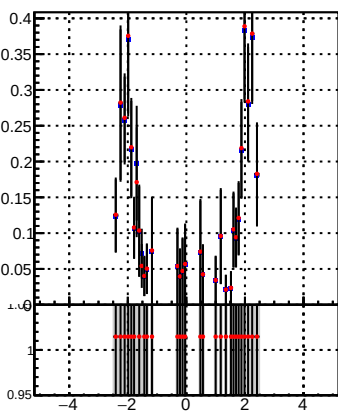
p_offset_eta_npv32_lep
