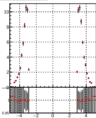
p_offset_eta_npv32_hfe
