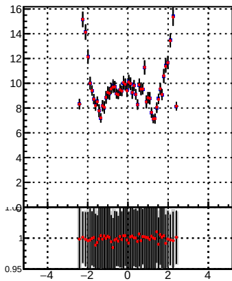
p_offset_eta_npv32_chm
