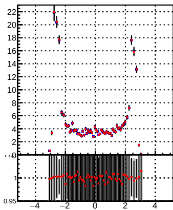
p_offset_eta_npv32_chu
