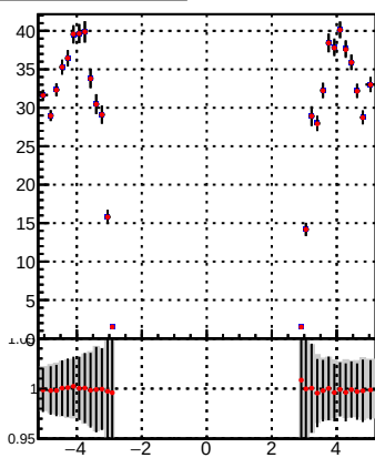
p_offset_eta_npv32_hfh
