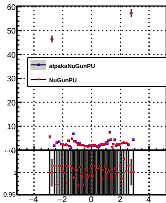
p_offset_eta_npv32_nh
