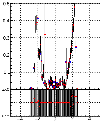
p_offset_eta_npv42_lep
