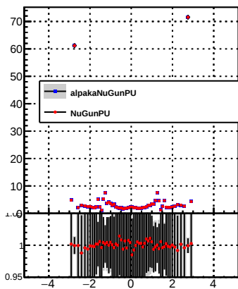
p_offset_eta_npv42_nh
