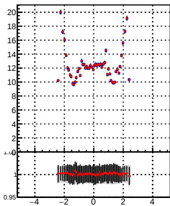
p_offset_eta_npv42_chm
