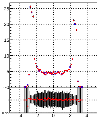
p_offset_eta_npv42_chu
