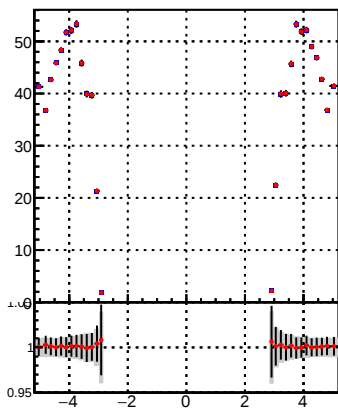
p_offset_eta_npv42_hfh
