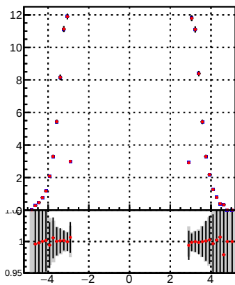
p_offset_eta_npv42_hfe
