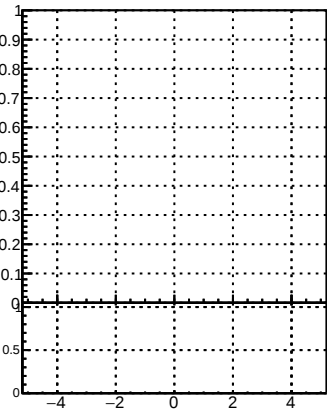
p_offset_eta_npv90_lep
