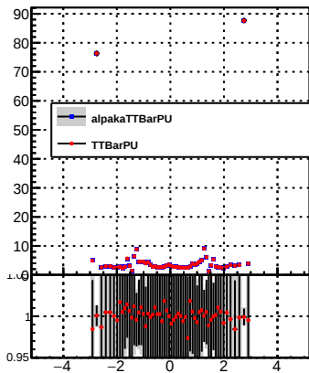
p_offset_eta_npv50_nh
