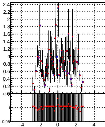
p_offset_eta_npv50_lep
