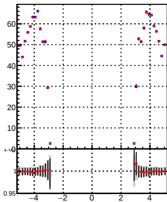
p_offset_eta_npv50_hfh
