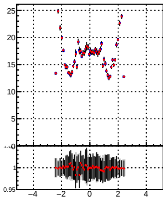
p_offset_eta_npv50_chm
