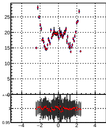
p_offset_eta_npv58_chm
