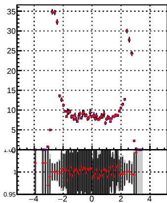
p_offset_eta_npv58_chu
