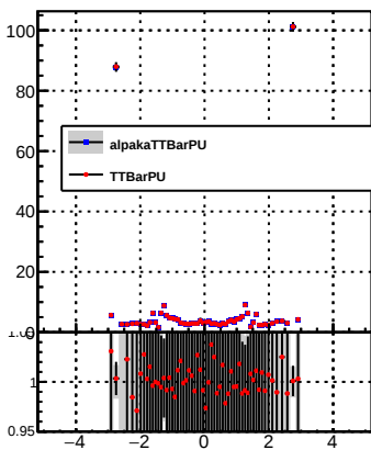
p_offset_eta_npv58_nh
