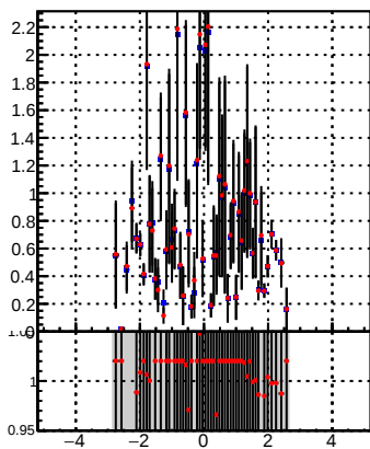
p_offset_eta_npv58_lep
