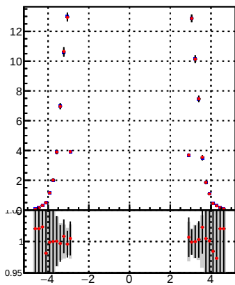
p_offset_eta_npv58_hfe
