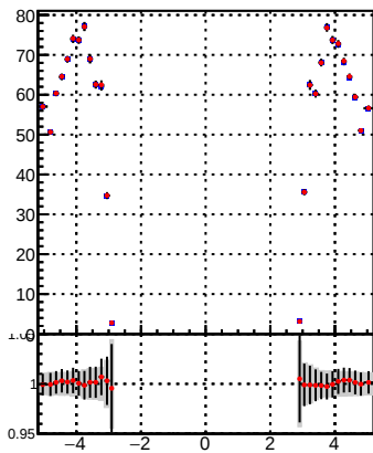
p_offset_eta_npv58_hfh
