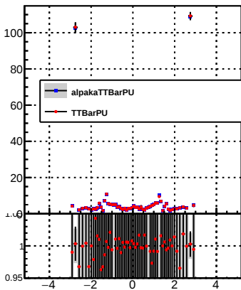
p_offset_eta_npv64_nh
