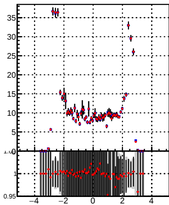
p_offset_eta_npv64_chu
