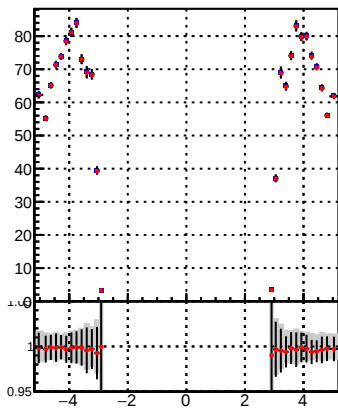
p_offset_eta_npv64_hfh
