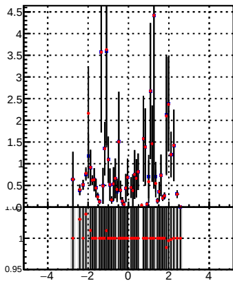
p_offset_eta_npv64_lep
