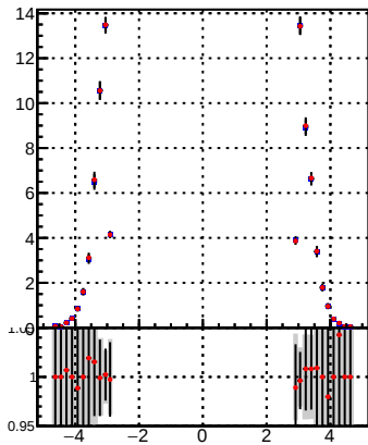
p_offset_eta_npv64_hfe
