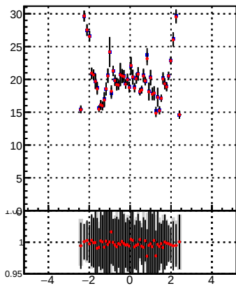
p_offset_eta_npv64_chm
