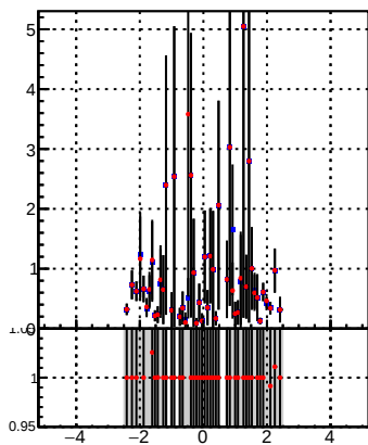
p_offset_eta_npv67_lep
