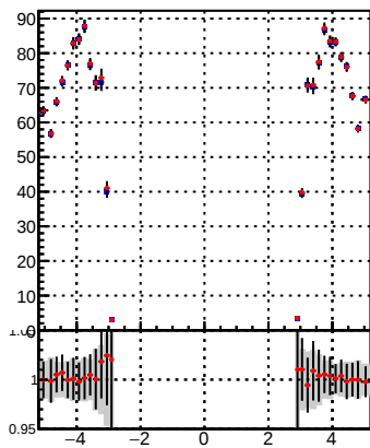
p_offset_eta_npv67_hfh
