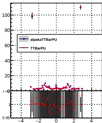
p_offset_eta_npv67_nh
