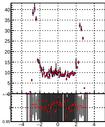
p_offset_eta_npv67_chu
