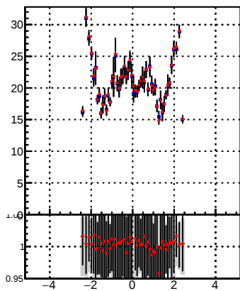
p_offset_eta_npv67_chm
