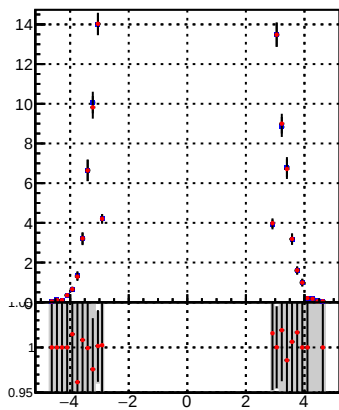
p_offset_eta_npv67_hfe
