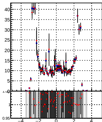
p_offset_eta_npv73_chu
