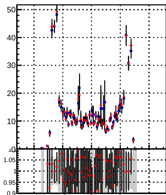
p_offset_eta_npv77_chu
