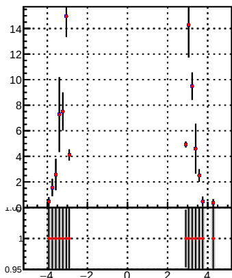
p_offset_eta_npv80_hfe
