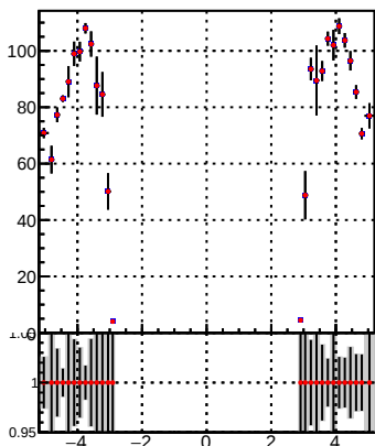
p_offset_eta_npv80_hfh
