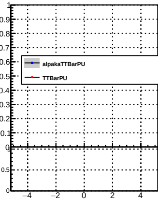
p_offset_eta_npv96_nh
