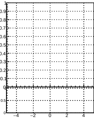
p_offset_eta_npv96_hfh
