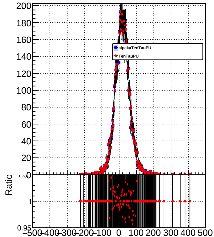
METDifference_GenMETTrue
