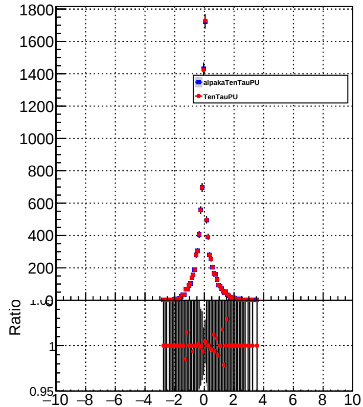
METUnc_ElectronEnDown
