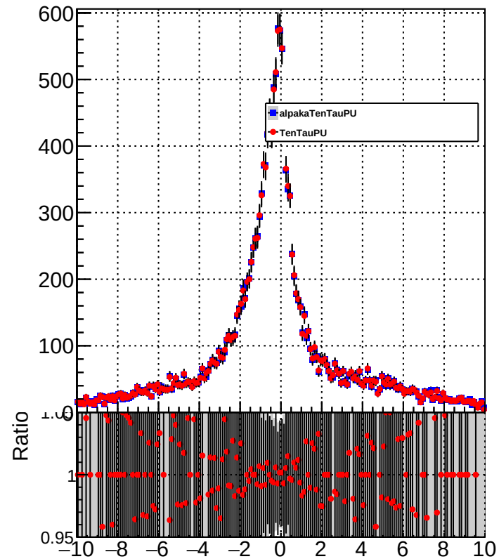
METUnc_UnclusteredEnDown
