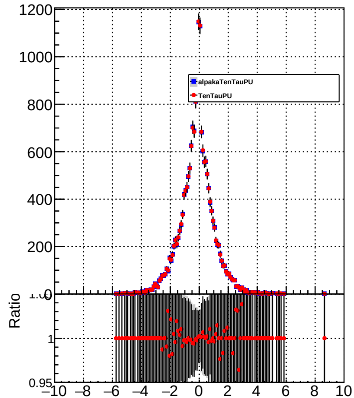
METUnc_UnclusteredEnDown
