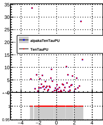
p_offset_eta_npv18_nh
