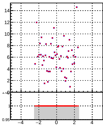
p_offset_eta_npv18_chm
