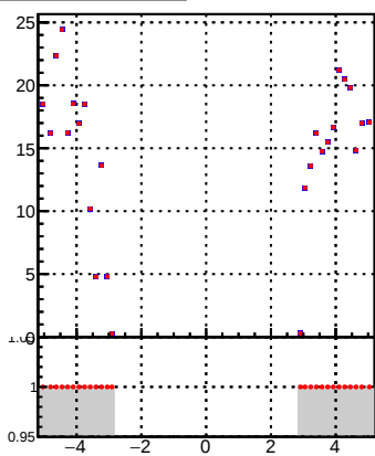
p_offset_eta_npv18_hfh
