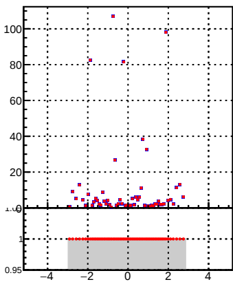
p_offset_eta_npv18_chu
