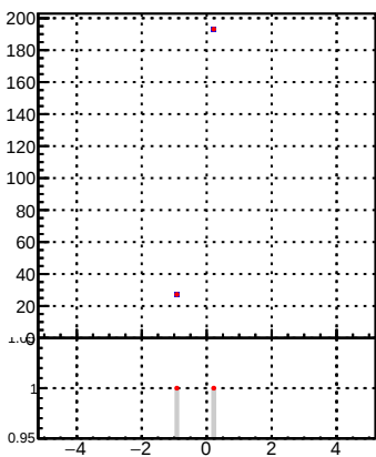
p_offset_eta_npv18_lep
