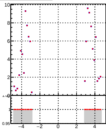
p_offset_eta_npv18_hfe
