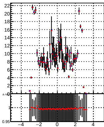
p_offset_eta_npv35_chu
