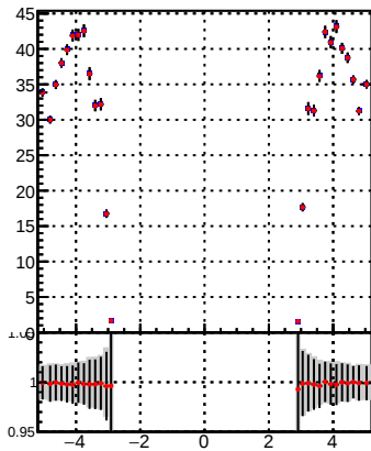
p_offset_eta_npv35_hfh
