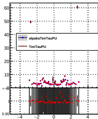
p_offset_eta_npv35_nh
