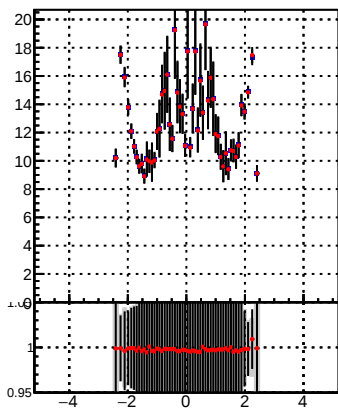
p_offset_eta_npv35_chm
