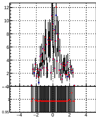
p_offset_eta_npv35_lep
