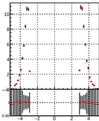
p_offset_eta_npv35_hfe
