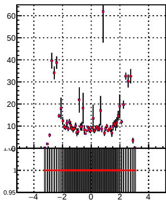
p_offset_eta_npv73_chu
