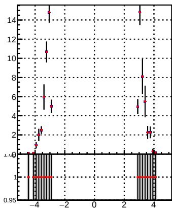
p_offset_eta_npv73_hfe
