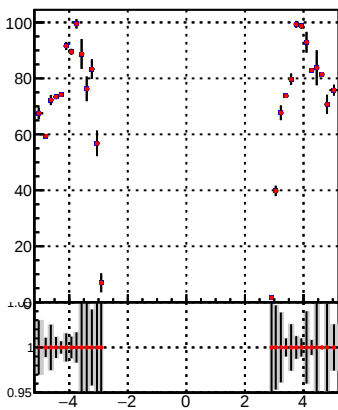
p_offset_eta_npv75_hfh
