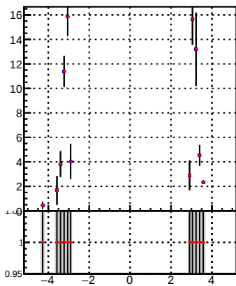
p_offset_eta_npv75_hfe
