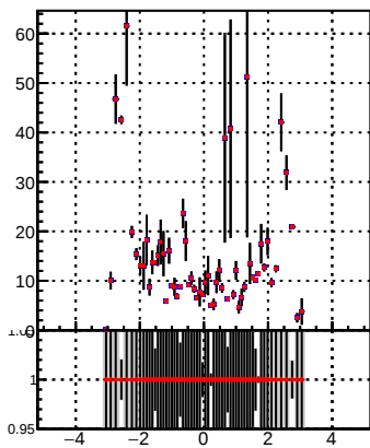
p_offset_eta_npv75_chu
