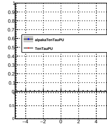
p_offset_eta_npv86_nh
