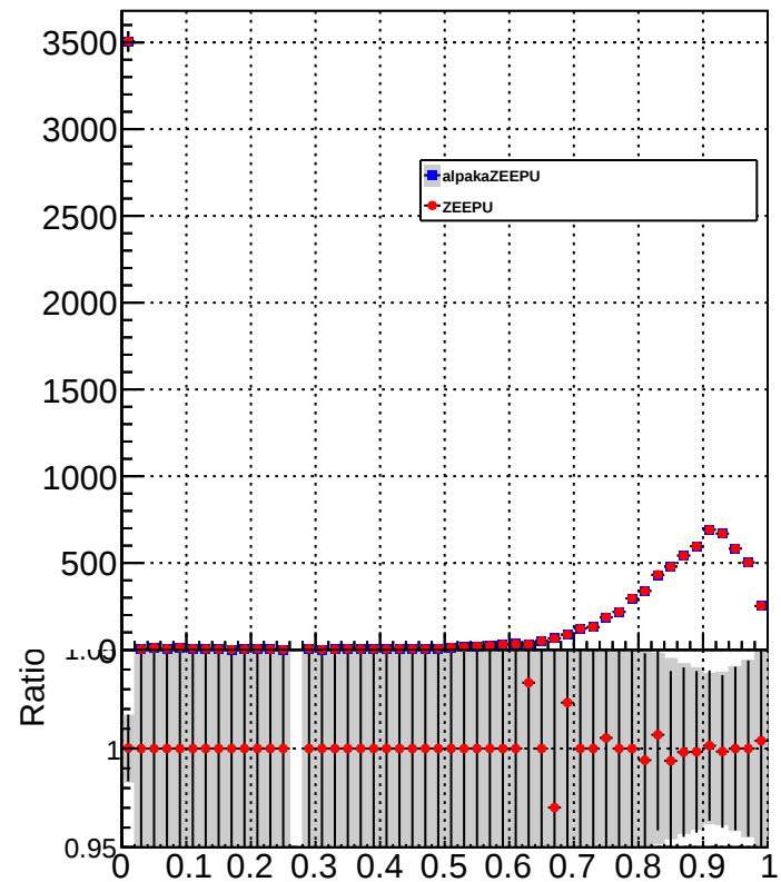
chargedEmEnergyFraction
