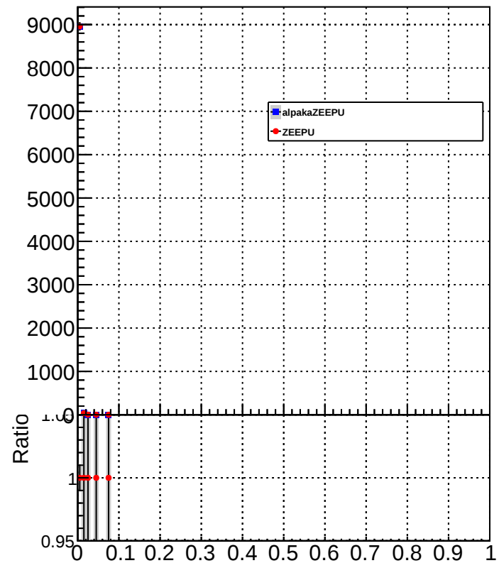
muonEtFraction
