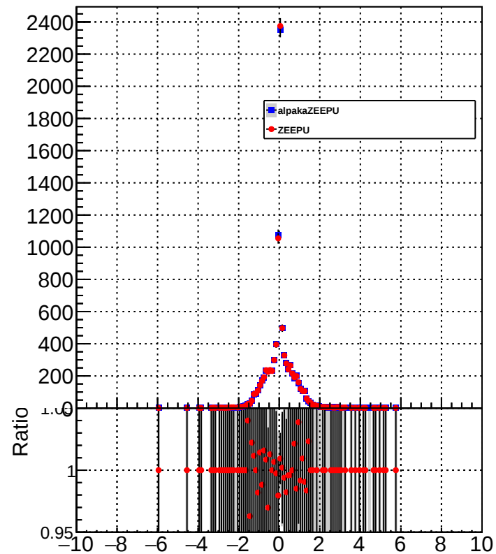
METUnc_TauEnDown
