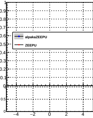
p_offset_eta_npv0_nh
