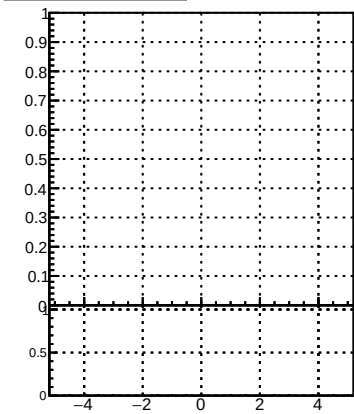
p_offset_eta_npv14_chu
