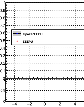
p_offset_eta_npv25_nh
