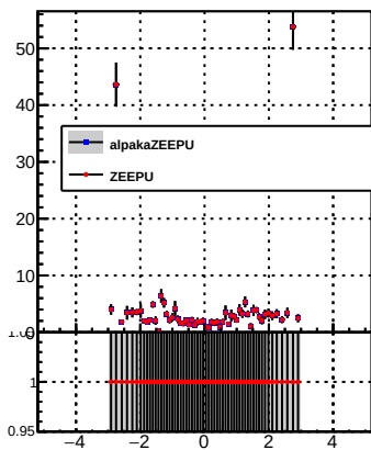
p_offset_eta_npv29_nh
