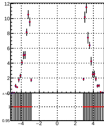
p_offset_eta_npv29_hfe
