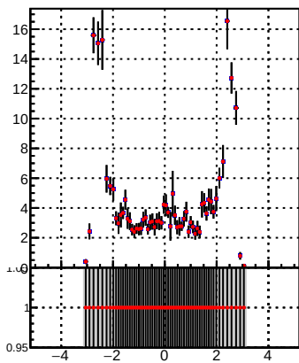
p_offset_eta_npv29_chu
