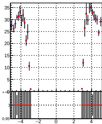
p_offset_eta_npv29_hfh
