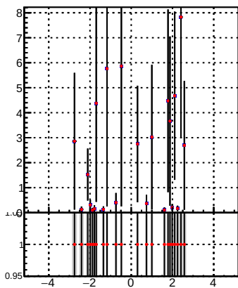
p_offset_eta_npv29_lep
