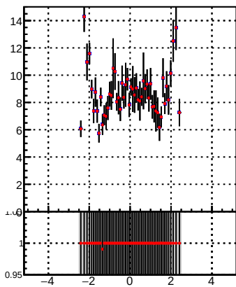
p_offset_eta_npv29_chm
