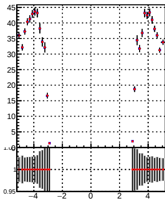
p_offset_eta_npv33_hfh
