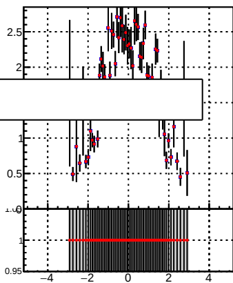
p_offset_eta_npv33_ne
