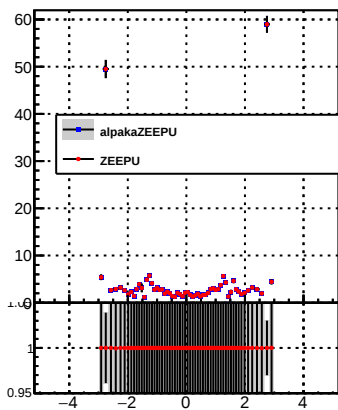
p_offset_eta_npv33_nh
