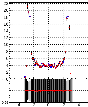
p_offset_eta_npv33_chu
