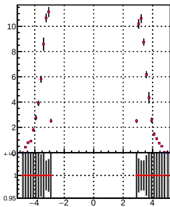
p_offset_eta_npv33_hfe
