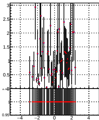
p_offset_eta_npv33_lep
