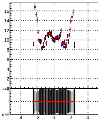
p_offset_eta_npv33_chm
