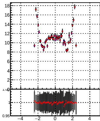
p_offset_eta_npv35_chm
