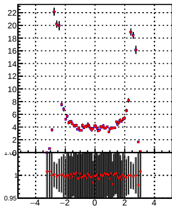
p_offset_eta_npv35_chu
