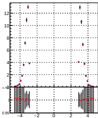
p_offset_eta_npv60_hfe
