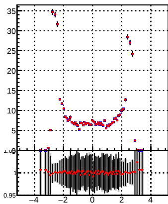
p_offset_eta_npv60_chu
