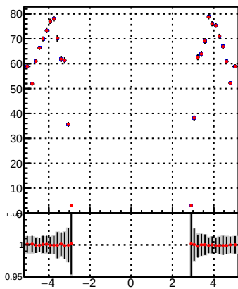
p_offset_eta_npv60_hfh
