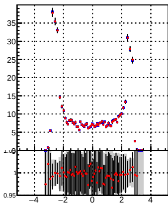
p_offset_eta_npv63_chu
