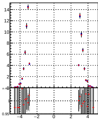
p_offset_eta_npv63_hfe
