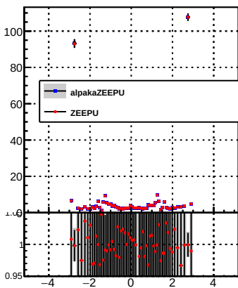
p_offset_eta_npv63_nh
