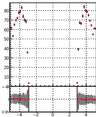
p_offset_eta_npv63_hfh
