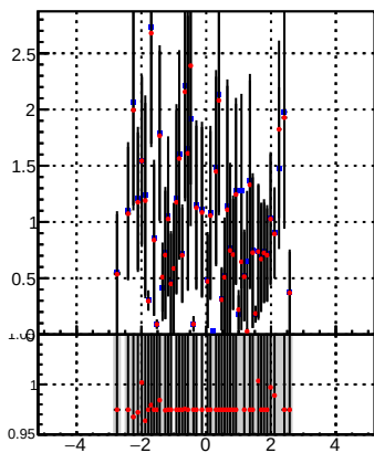
p_offset_eta_npv63_lep
