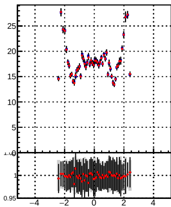
p_offset_eta_npv63_chm
