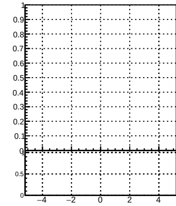
p_offset_eta_npv88_hfh
