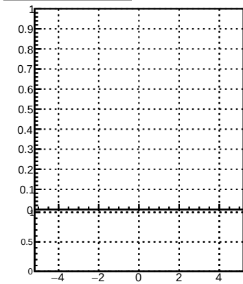
p_offset_eta_npv88_chm
