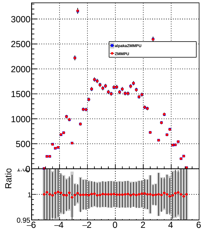
CorrJetEta Pt>20
